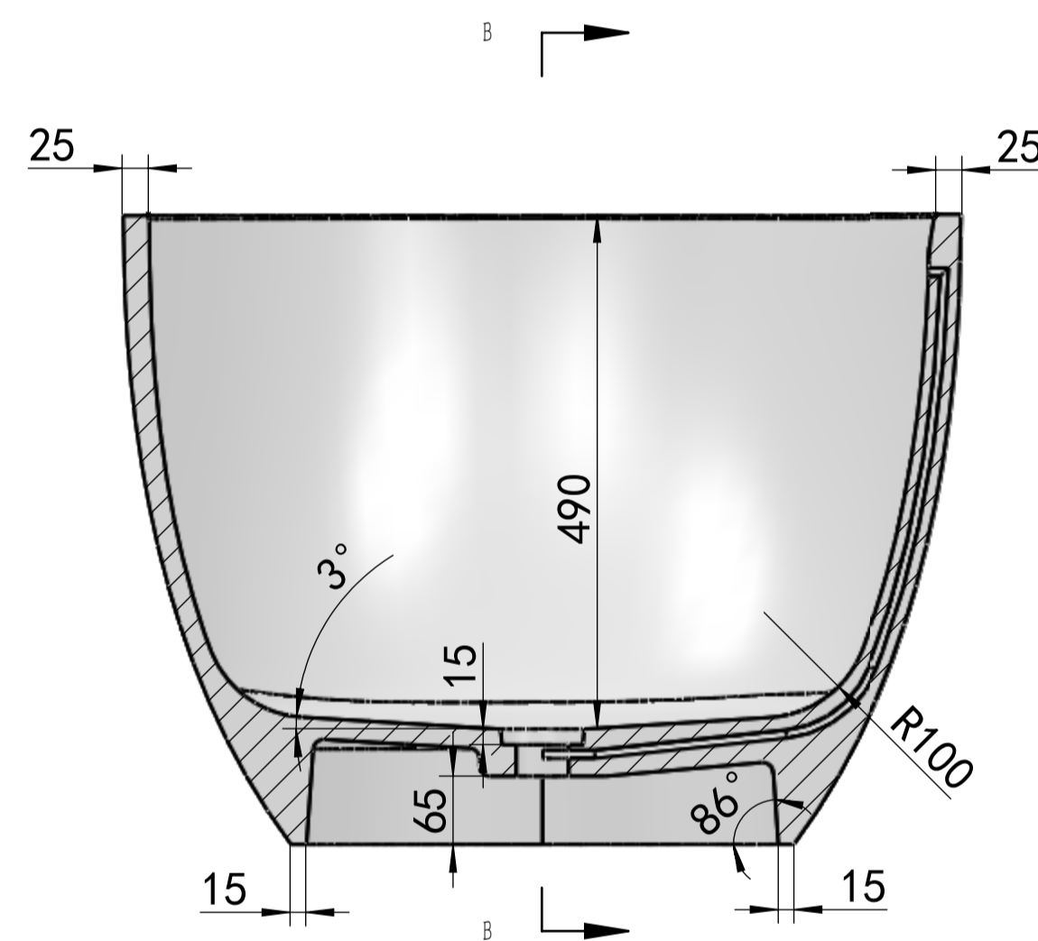
A-A 1 : 6.5
